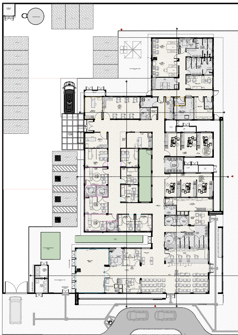
PLANTA DE LAYOUT F01115
