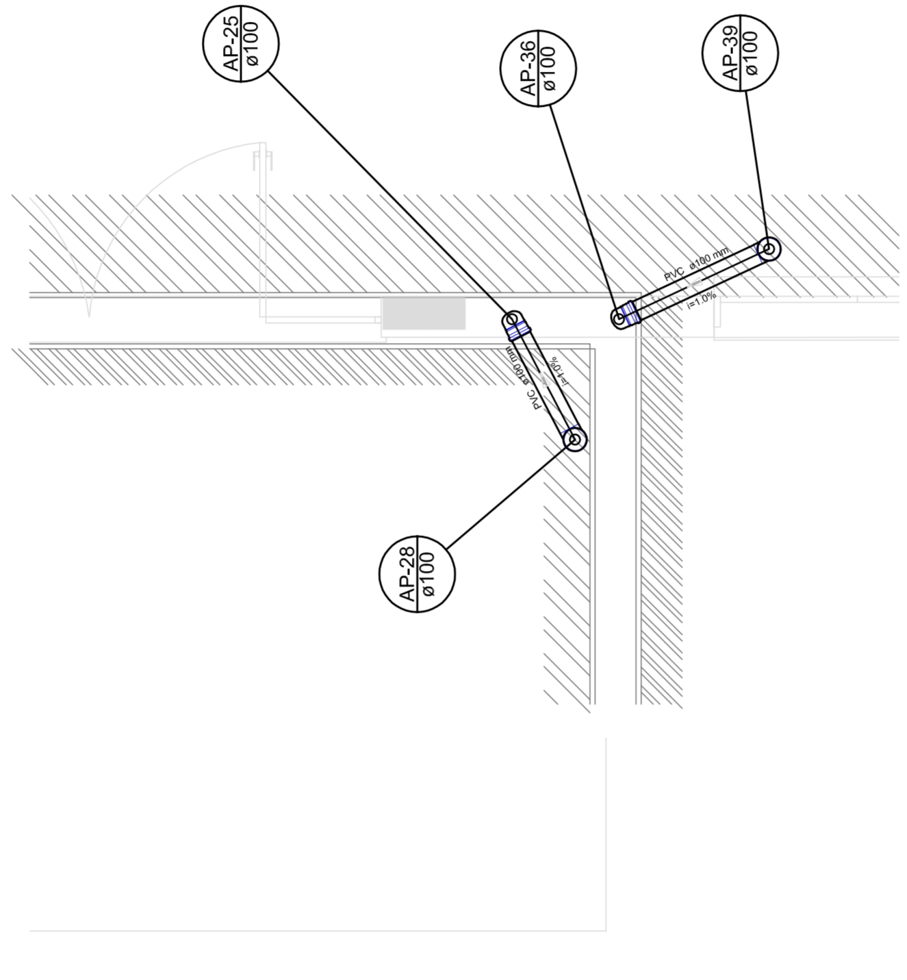
Detalle S7 escala 1:25
